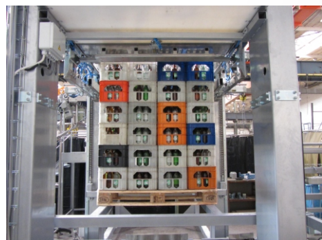
NMP 1500 - подъемник паллет
