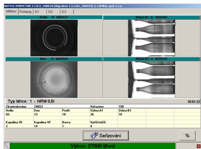
Exan 08 CCD - Einstellpanel
