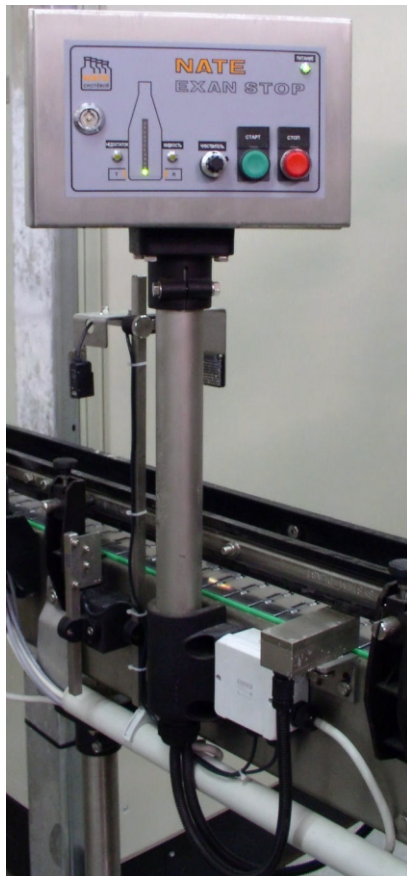
Exan Stop (Kontrolle der Restflüssigkeiten vor dem Füllen)
