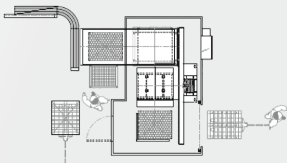
NMD 1000 P - Al Ain Mineral Water Company, Объединенные Арабские Эмираты
